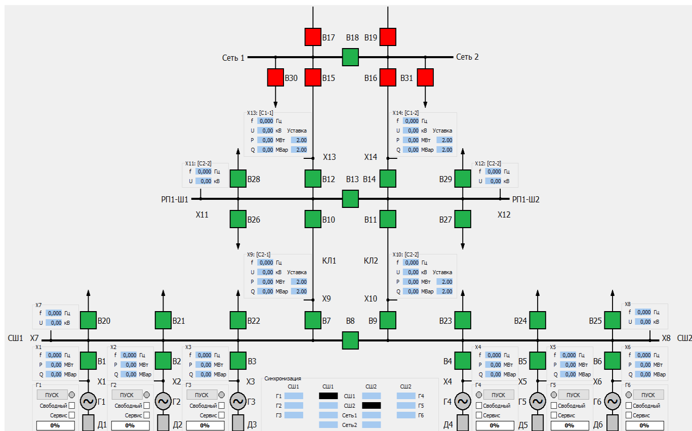
Рисунок И.1 – Видеоквадр симулятора со схемой ЛИЭС
