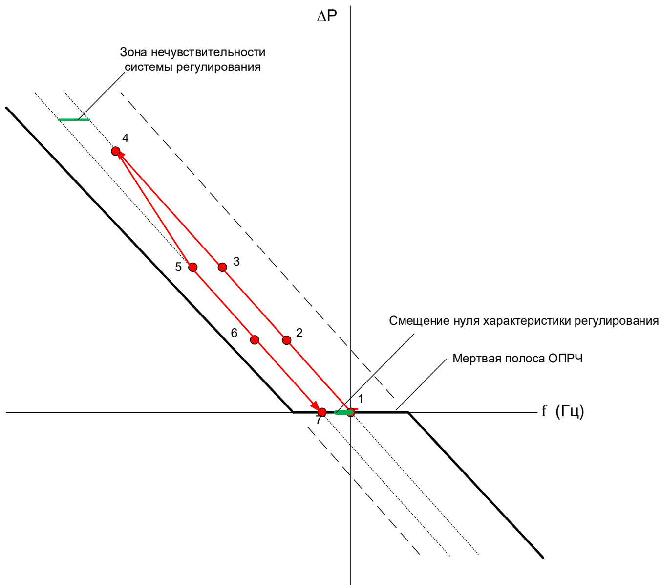
Рисунок С.1 – Характеристики ОПРЧ и иллюстрация методики определения K_s , зоны нечувствительности и смещения характеристик
