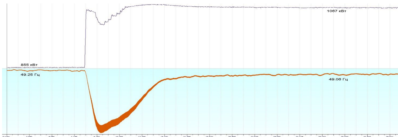
Рисунок С.9 – Включение ВТЭН1,2
