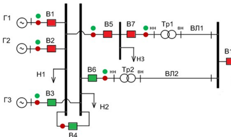
Рисунок Н.1 – Схема испытательной установки и внешний вид физической модели ЭС
