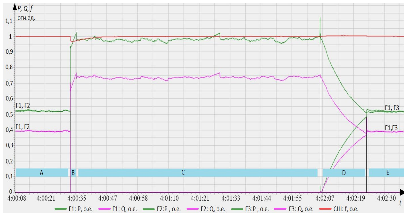
Рисунок И.7 – График процесса при аварийном отключении ЛИЭС от внешней сети (интервал с первого по шестой часе суточного графика)
