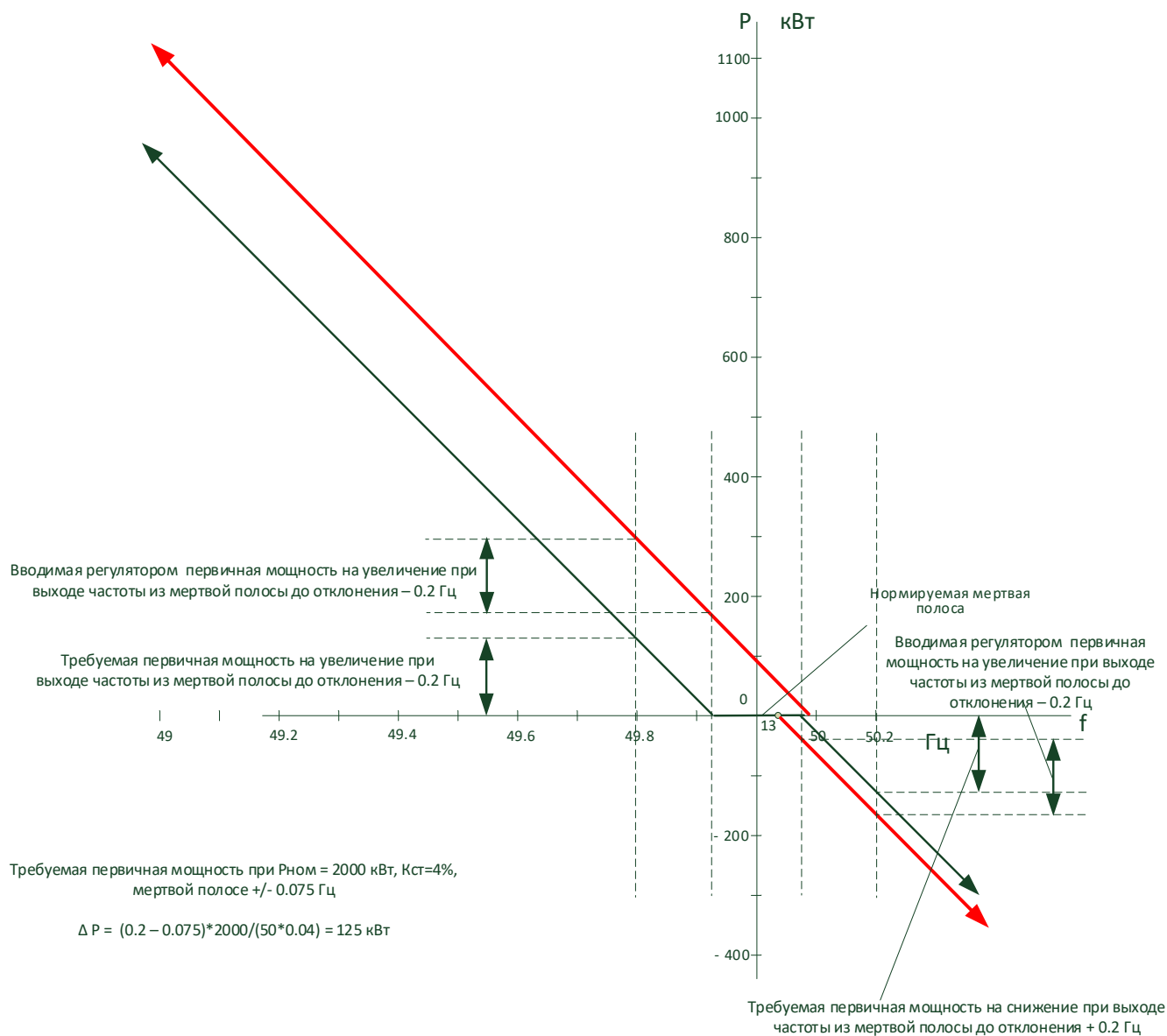
Рисунок С.17 – Подтверждение реализации требуемой первичной мощности генератором Г5
