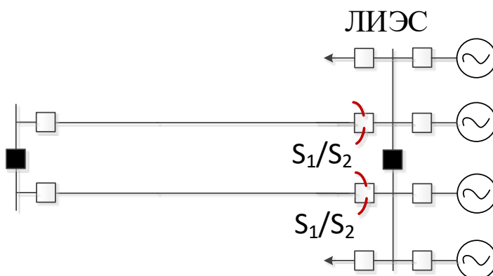
Рисунок А.2 – Базовая схема присоединения к ПС внешней электрической сети ТЭС ЛИЭС с разделяющей на две симметричные части без РП
