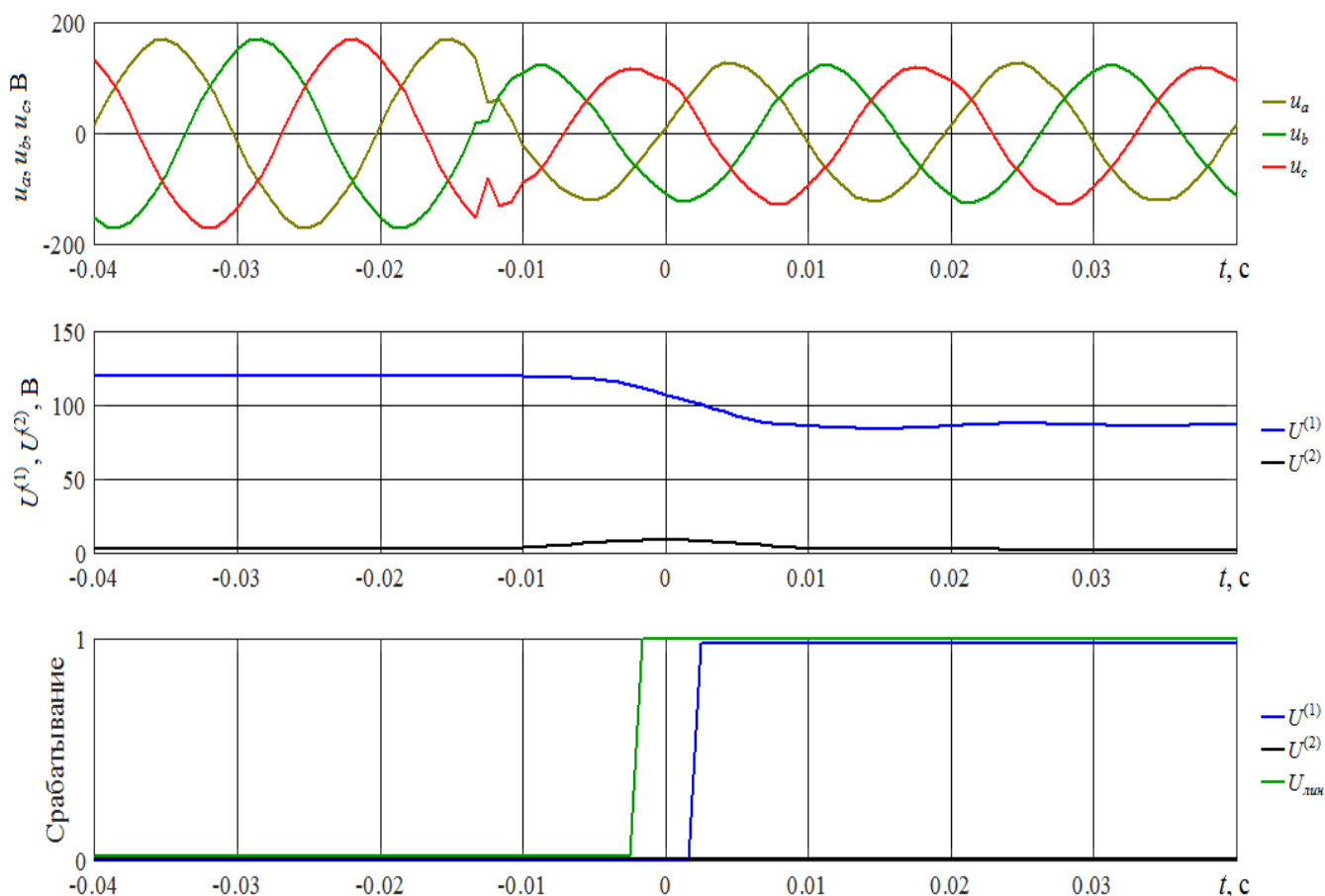
Рисунок Н.2 – Осциллограмма напряжений в фазах (верхняя часть), напряжения прямой и обратной последовательностей (средняя часть), сигналы срабатывания по каналам
